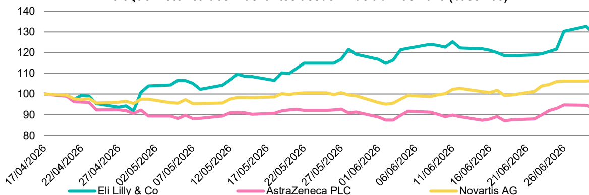
Evolução histórica dos indexantes desde 17 de abril de 2026 (base 100)
